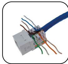
Accommodate the eight wires on the jack Acomoda los ocho cables en el conector
